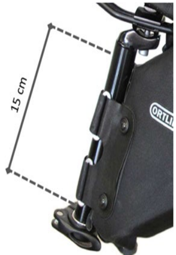
Erforderlicher Abstand für die Montage des Seat-Pack Limited Edition 16,5 L an der Sattelstütze
